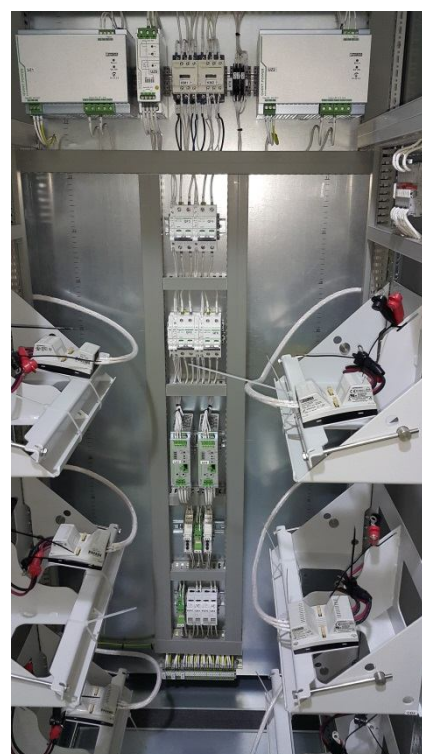
Рисунок 2 – организация бесперебойного питания с помощью серии Quint
